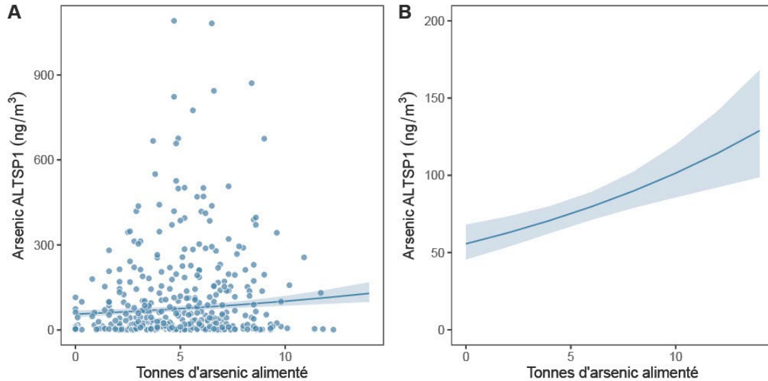
Figure 3. Relation entre la quantité journalière d'arsenic alimentée au réacteur de la Fonderie Horne et la concentration journalière en arsenic à la station ALTSP1 (A). La ligne continue représente la prédiction du modèle, et la surface ombragée représente l'intervalle de confiance à 95 % autour de la prédiction, alors que les points représentent les valeurs mesurées. Les prédictions seules (B) sont présentées afin de faciliter la visualisation des tendances.
