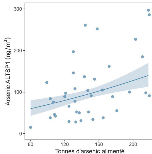
Figure 2. Relation entre la quantité mensuelle d'arsenic alimentée au réacteur de la Fonderie Horne et la concentration moyenne mensuelle en arsenic à la station ALTSP1. La ligne continue représente la prédiction du modèle, et la surface ombragée représente l'intervalle de confiance à 95 % autour de la prédiction, alors que les points représentent les valeurs mesurées.
