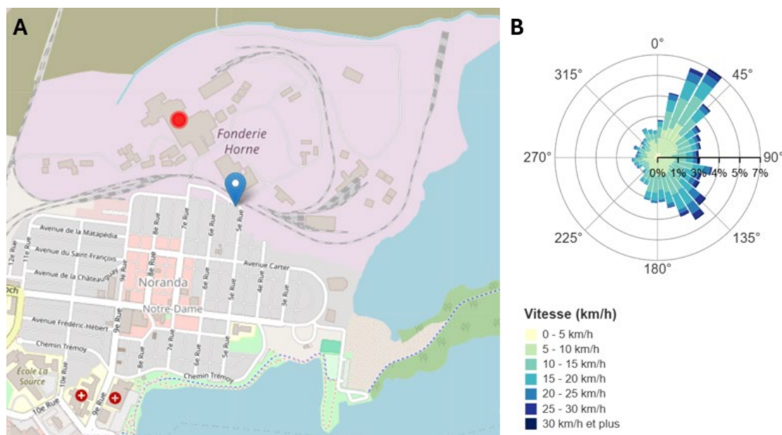
Figure 1. (A) Position de la station ALTSP1 (épingle bleue) par rapport au secteur du réacteur de la Fonderie Horne (point rouge). (B) Rose des vents illustrant la direction vers laquelle soufflent les vents ainsi que leur vitesse pour la période de janvier 2018 à juin 2021.
